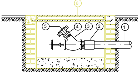
CORTE A-A
