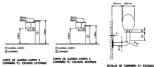
DETALHE DE CORRIMÃO P/ ESCADAS
