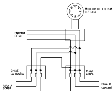
ESQUEMA - LIGAÇÃO DA BOMBA ELÉTRICA
