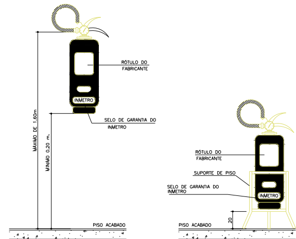
DETALHE TÍPICO DA INSTALAÇÃO DE EXTINTORES MANUAIS
