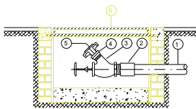
CORTE A-A
