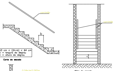
DETALHE DE CORRIMÃO P/ ESCADAS
