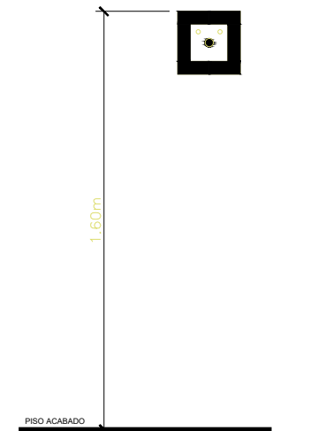
DETALHE DA INSTALAÇÃO DO ALARME
